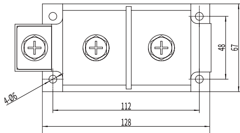
■ RH801600DA系列尺寸图
