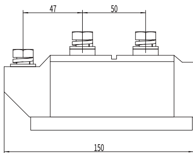
■ RH801200DA系列尺寸图
