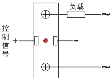
■ 150A-400A电流接线图
