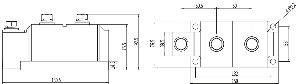
■ RH801600DA系列尺寸图
