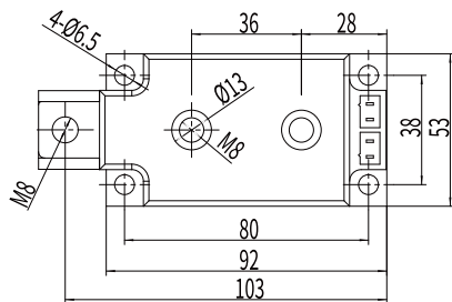
■ RH80800DA、801000DA系列尺寸图
