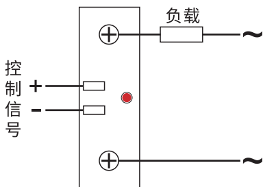
■ RH80系列接线图
