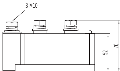
■ RH80800DA、801000DA系列尺寸图
