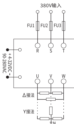
■ RG3系列电加热负载接线示意图
