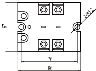
■ RG2系列尺寸图
