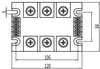
■ RG2系列尺寸图
