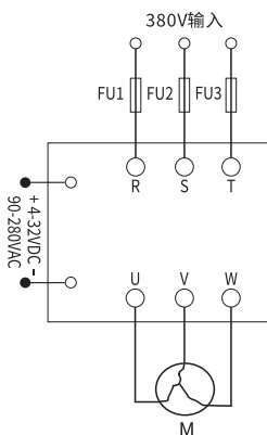
■ RG3系列电机类负载接线示意图
